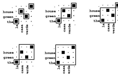
Figura 2. Posibles segmentaciones bilingües para una matriz de alineamiento a nivel de palabra dada.
